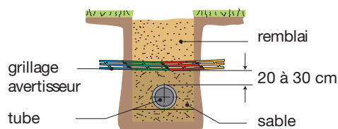
COUPE DE LA TRANCHÉE
