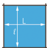
CARRÉE
