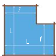
EN "L"
