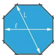
OCTOGONALE
