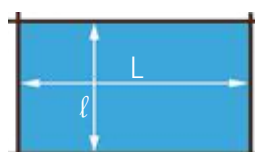
RECTANGULAIRE
