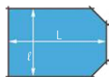
SEMI-OCTOGONALE
