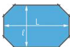
OCTOGONALE ALLONGÉE
